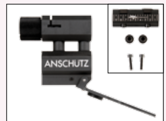
Kornstunnel Biathlon 6865 höhenverstellbar inkl. Visierlinienerhöhung um 8 mm. Biathlon front sight 6865 adjustable in height incl. rear sight elevation 8 mm. Art.-Nr.: 011360
